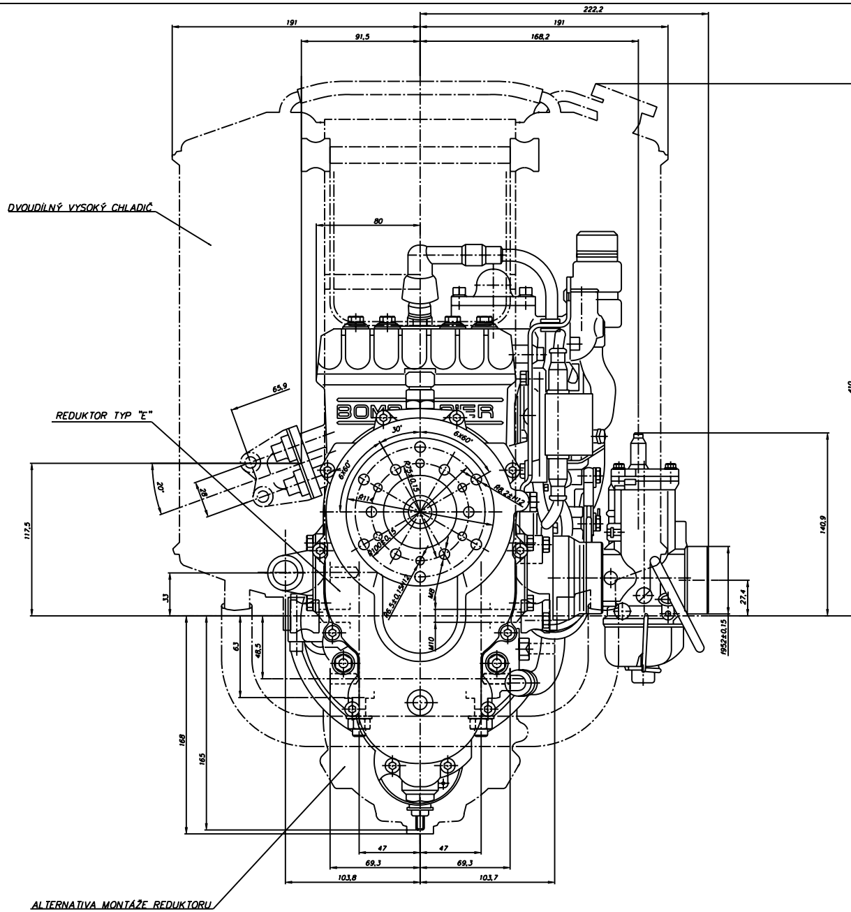
ROTAX 582 UL DCDI – POHLED OD VRTULE 582v.dxf
