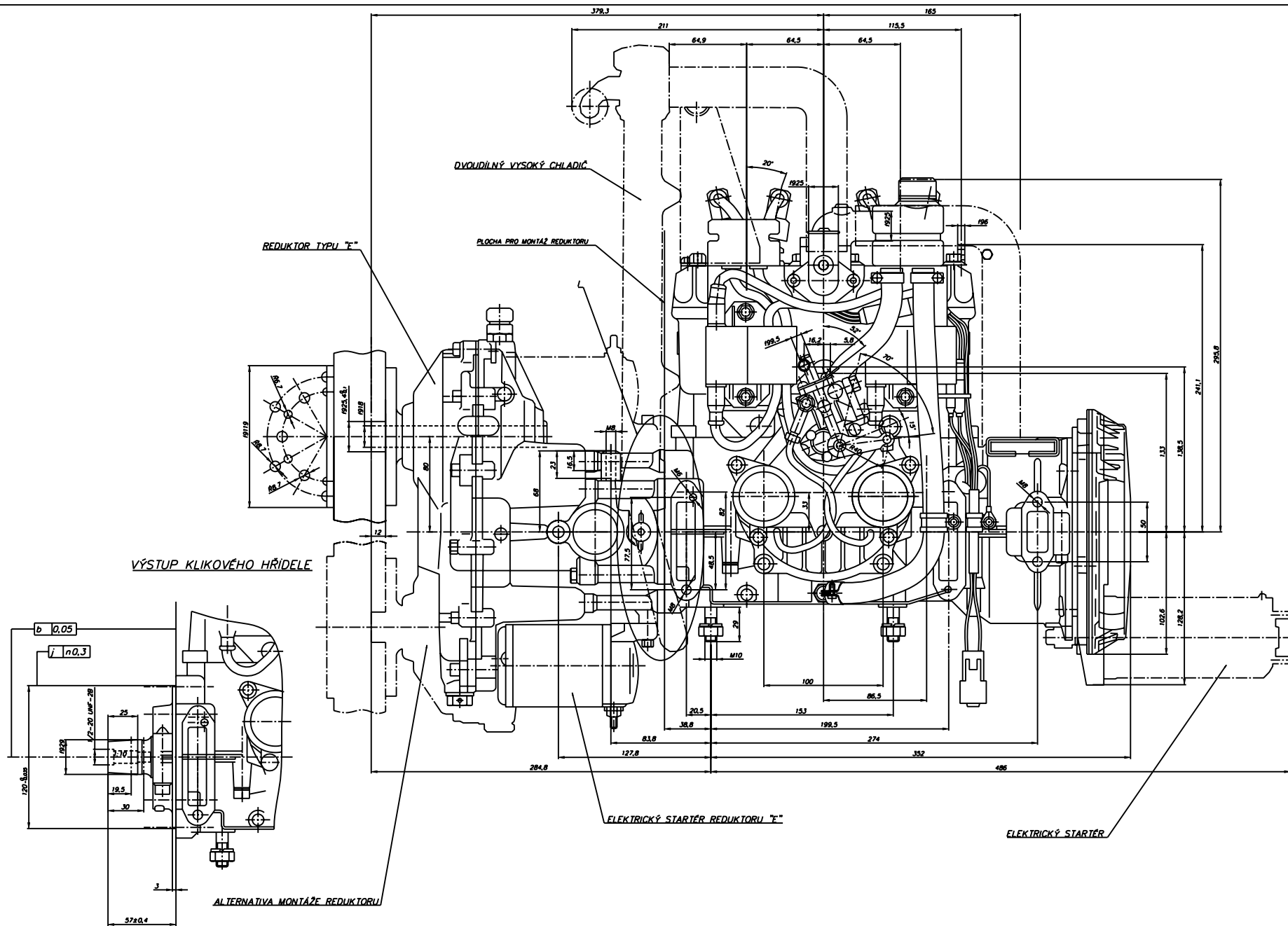
ROTAX 582 UL DCDI POHLED - Z BOKU 582b.dxf " pouze pro informaci "
