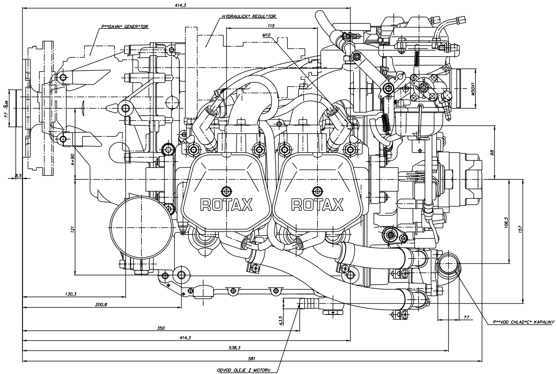
ROTAX 912 UL DCDI – POHLED Z BOKU 912b.dxf
