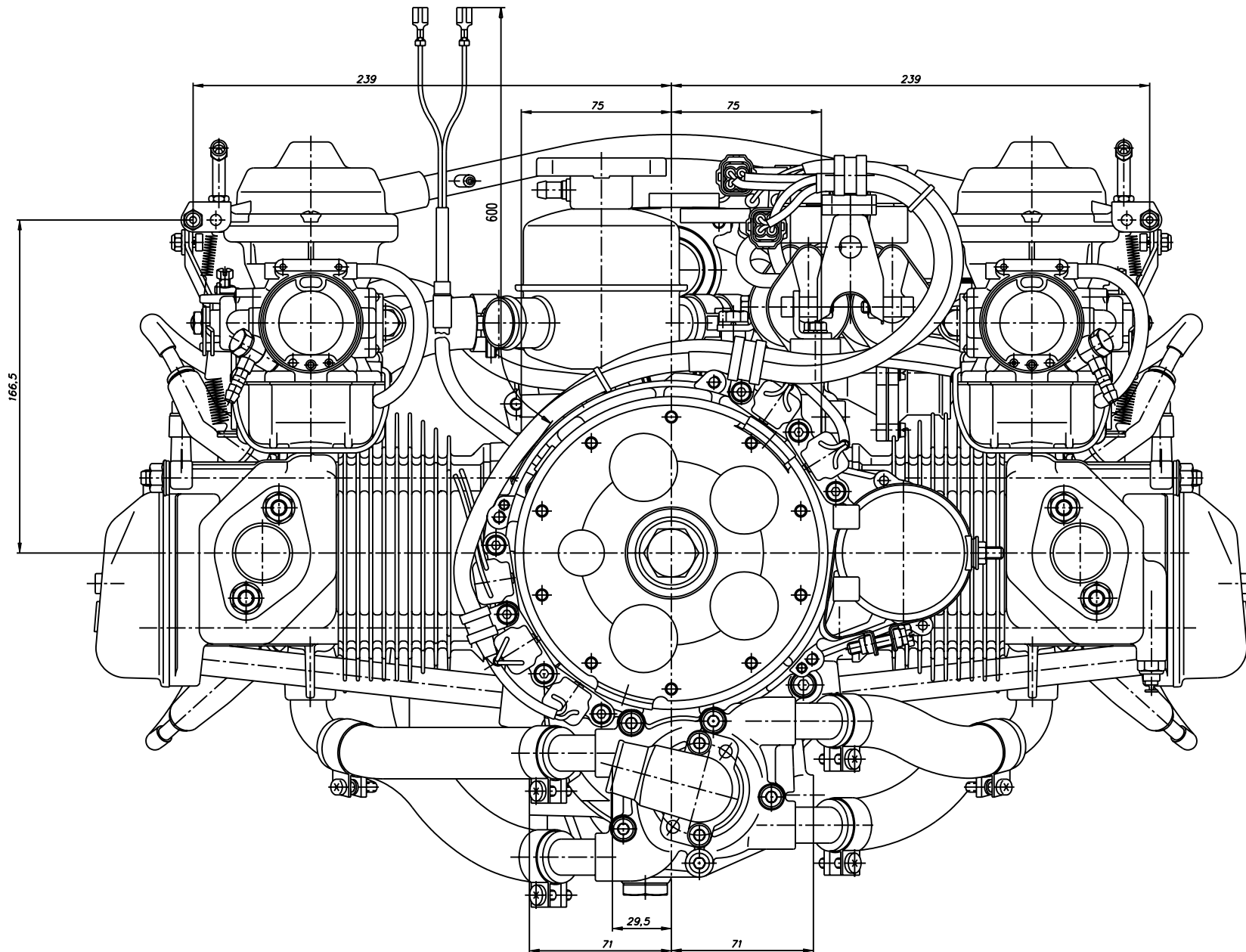
ROTAX 912 UL DCDI – POHLED OD GENERÁTORU 912g.dxf " pouze pro informaci "
