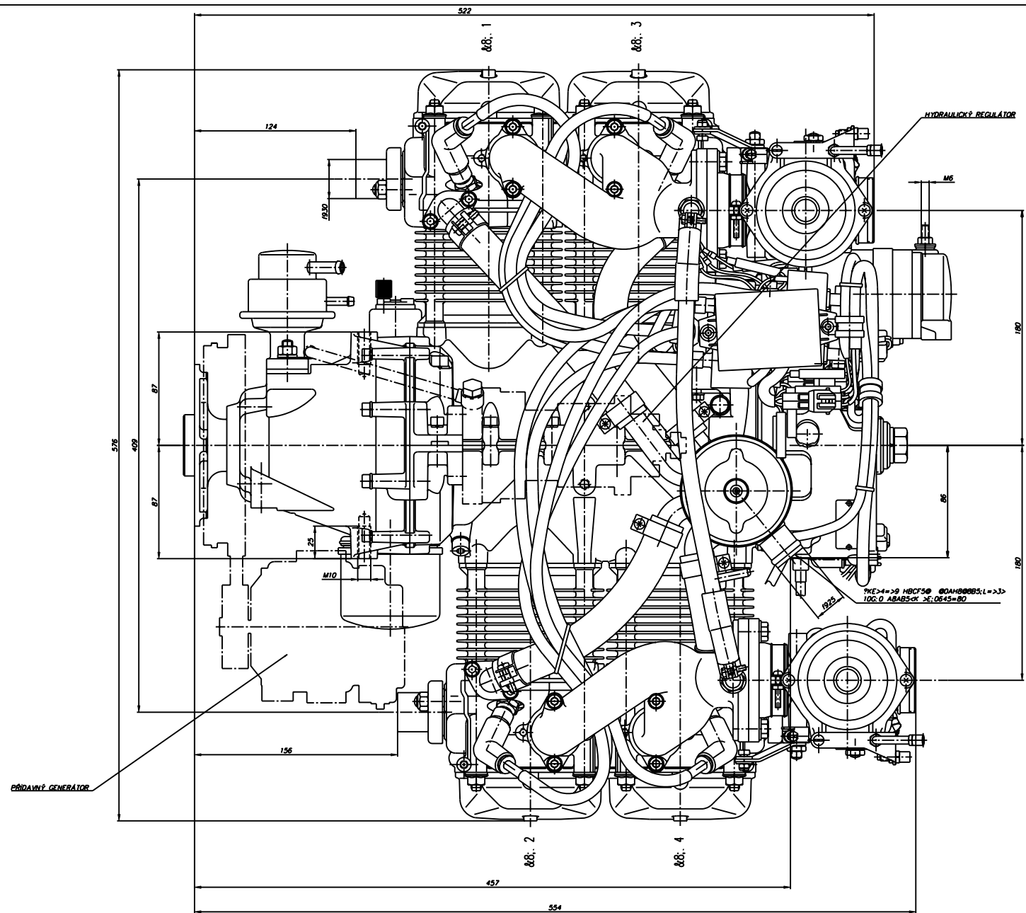
ROTAX 912 UL DCDI – POHLED ZE ZHORA 912z.dxf " pouze pro informaci "
