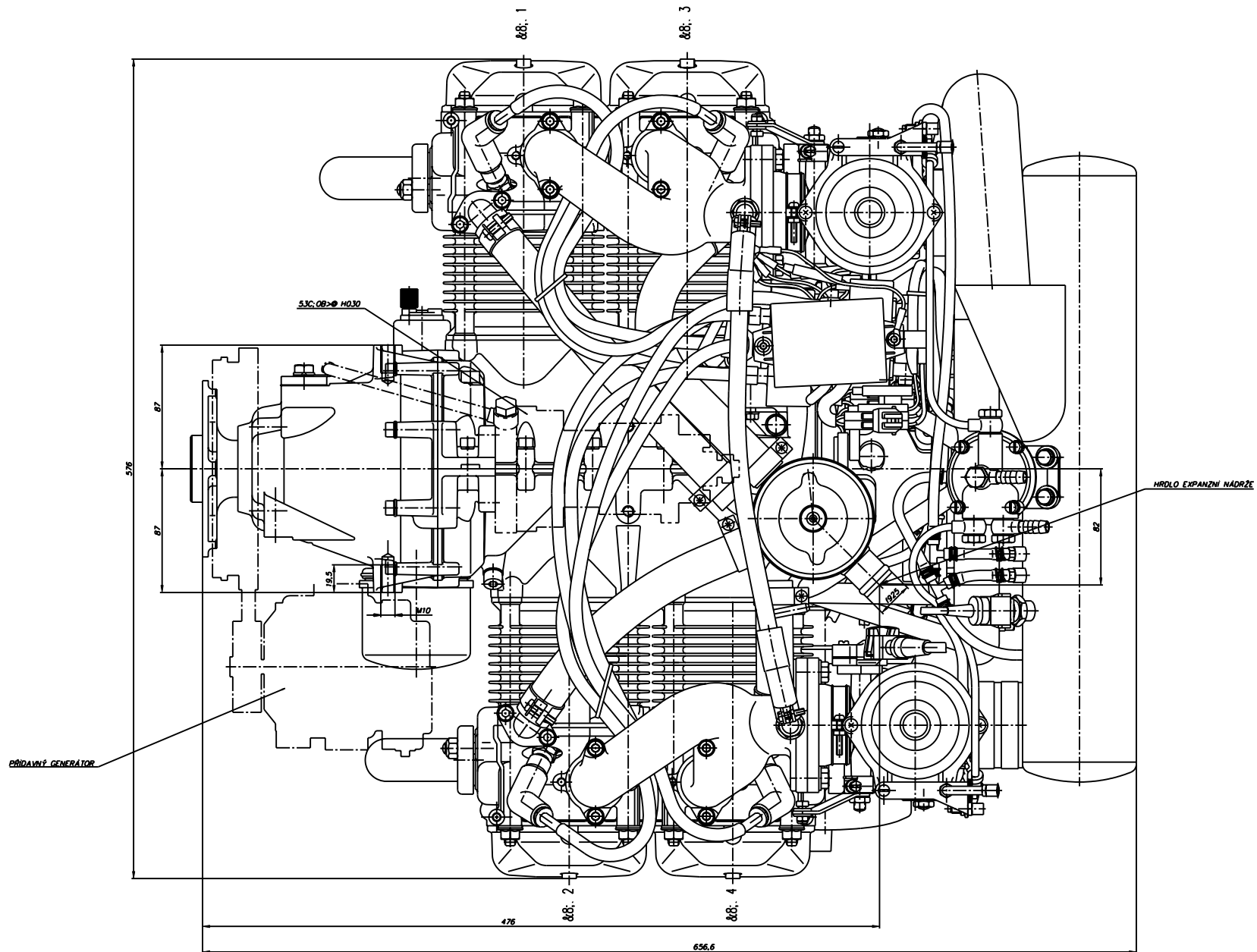
ROTAX 914 UL DCDI – POHLED ZE ZHORA 914z.dxf " pouze pro informaci "
